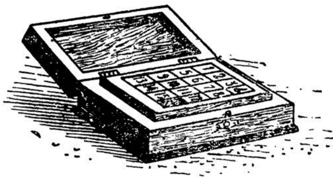
Рис. 13. Игра в 15.
