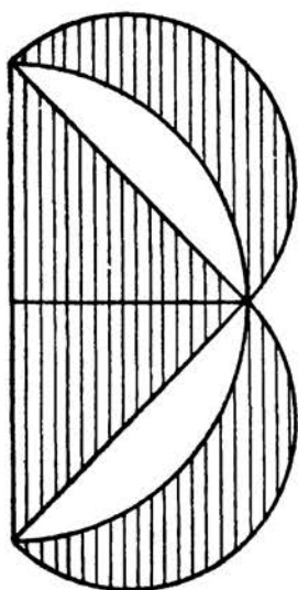
Рис. 154. Гиппократовы луночки.
