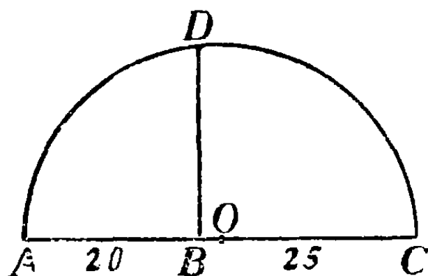
Черт. 29. Графическое извлечение квадратного корня.
